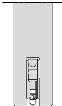
Automatische valdorpel
